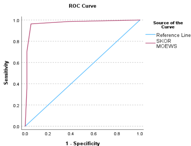
Gambar 1. Kurva ROC
