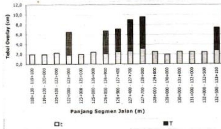
Disain Tebal Lapis Tambahan Yang Diperlukan (t dan T)
